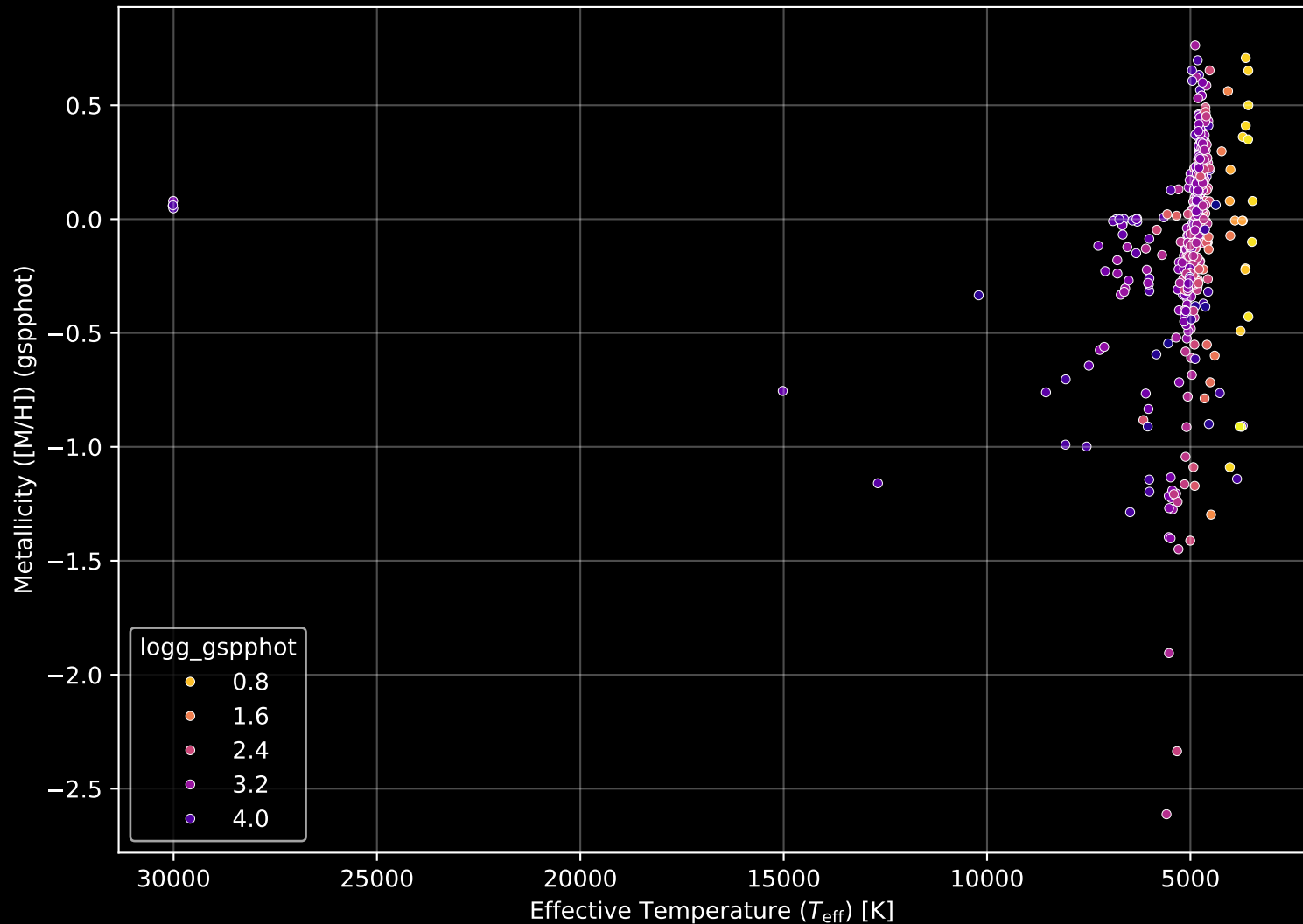
APOGEE DR17 Field: [020+04] Stellar Population Parameters (n= 564)
